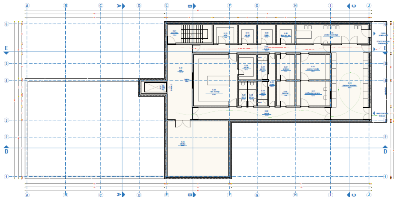
Slika 16: Tloris kleti
