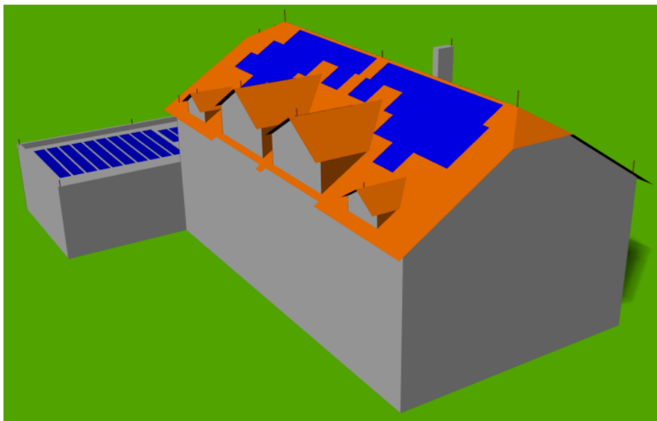
Pogled severovzhod: montirani paneli in LPS sistem: lovilne palice
