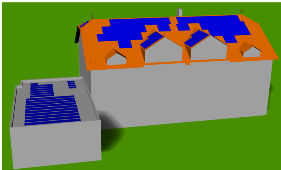
Pogled zahod: montirani paneli in LPS sistem: lovilne palice
